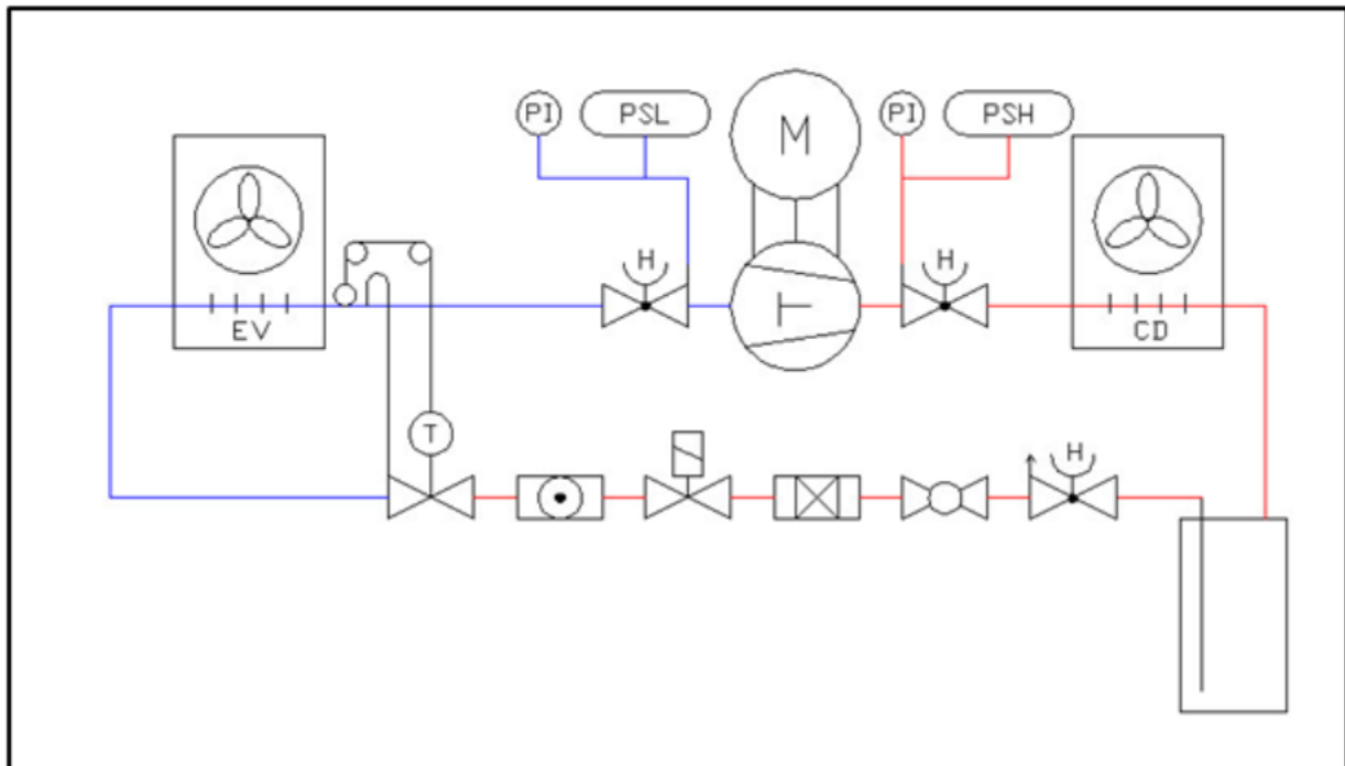
Exemple installation frigorifique
